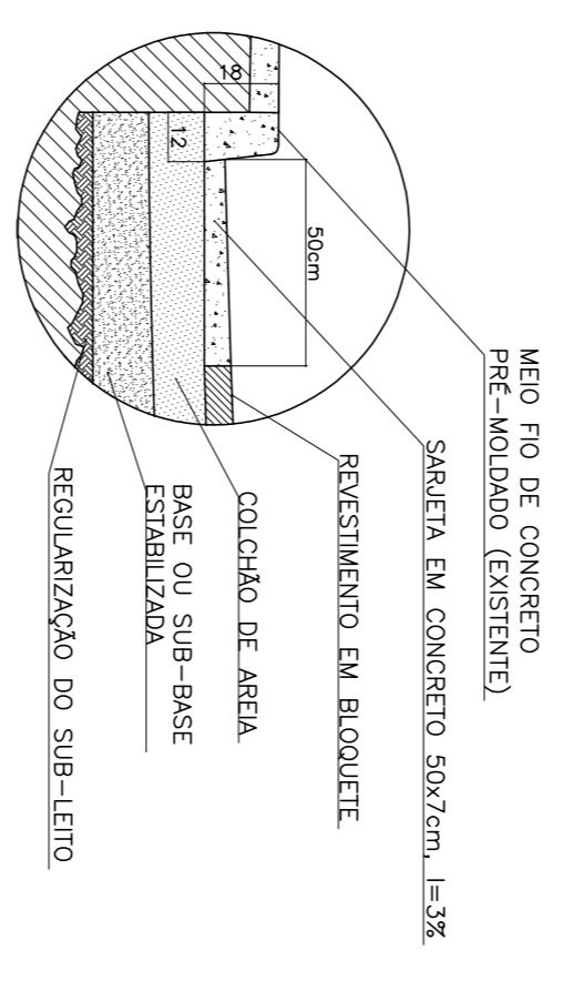
Detalle O1 Meio fio, sarjeta e bloquete
